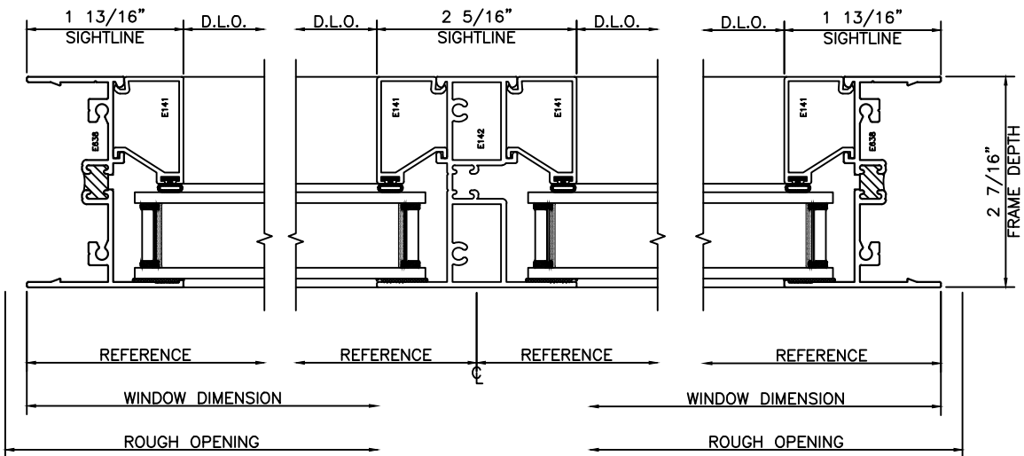
20 FIXED JAMB
