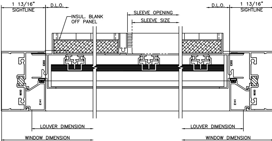
8 LOUVER JAMB
