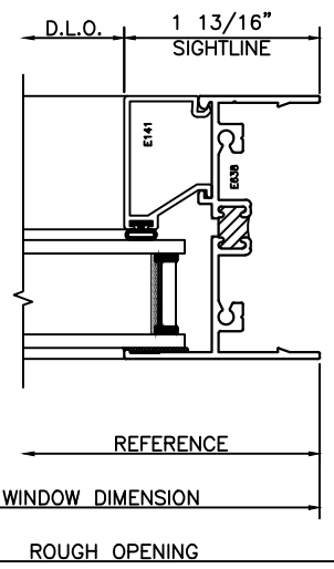
22 FIXED JAMB
